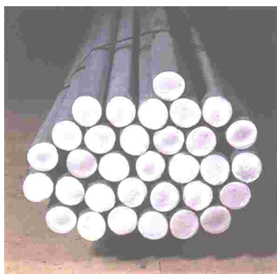
Barres de broyeur : Ø14mm à Ø100mm 37 HRC
