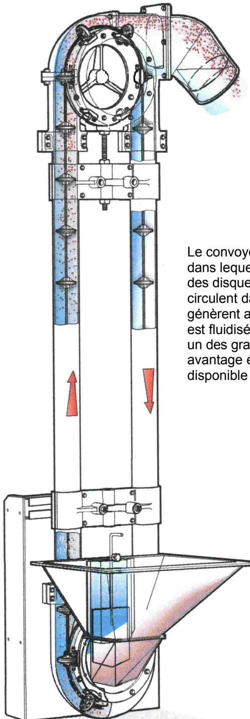
Tête convoyeur vertical avec vanne bippase
