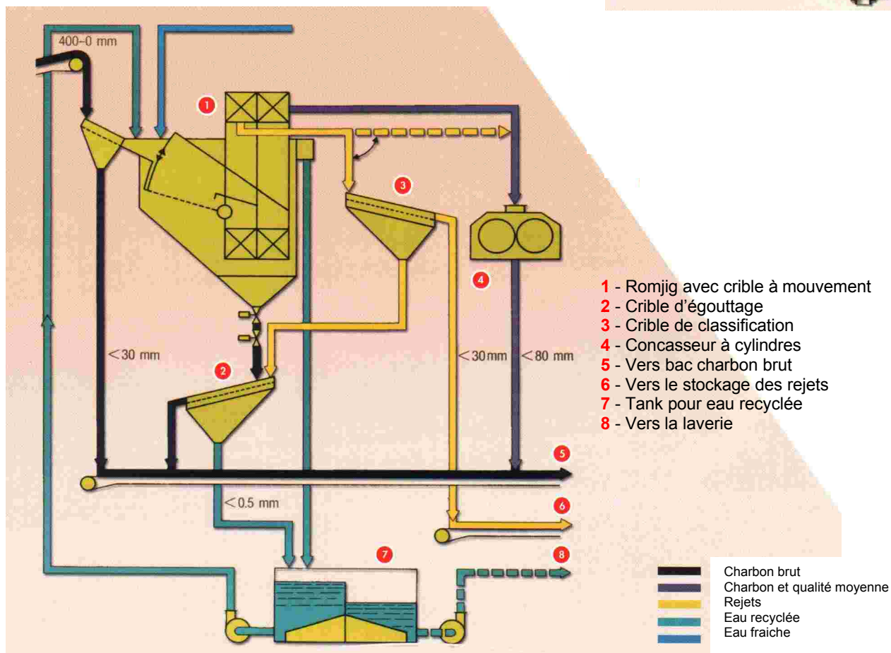
Séparation des rejets primaires avec le bac à pistonnage Romjig
